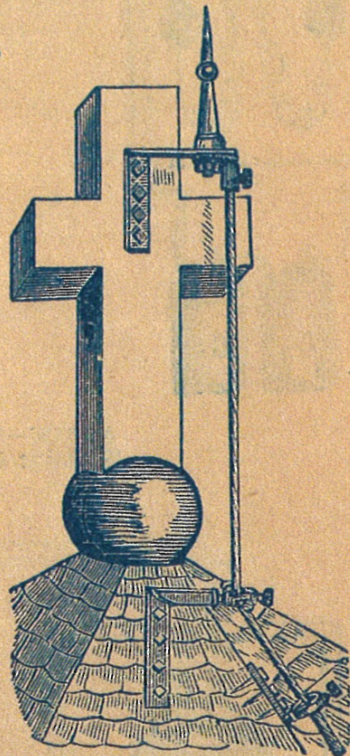
Torony-villámhárító. Kirchthurm-Blitzableiter.
