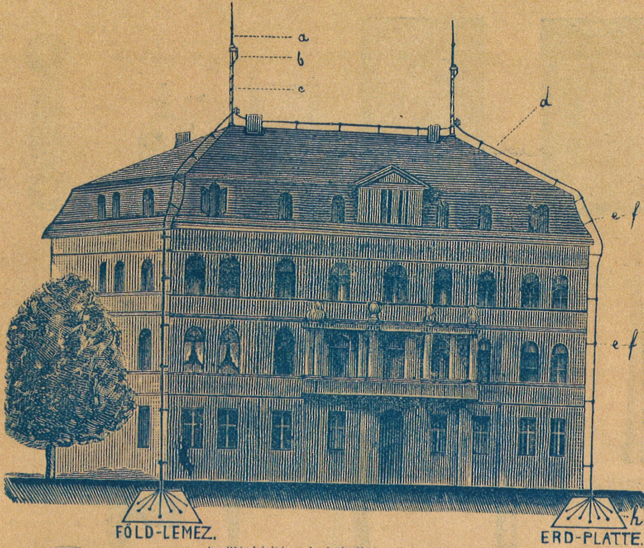
A villámhárító gyakorlati alkalmazása. 2601—2682. sz. Praktische Anwendung des Blitzableiters. Nr. 2601—2682.
