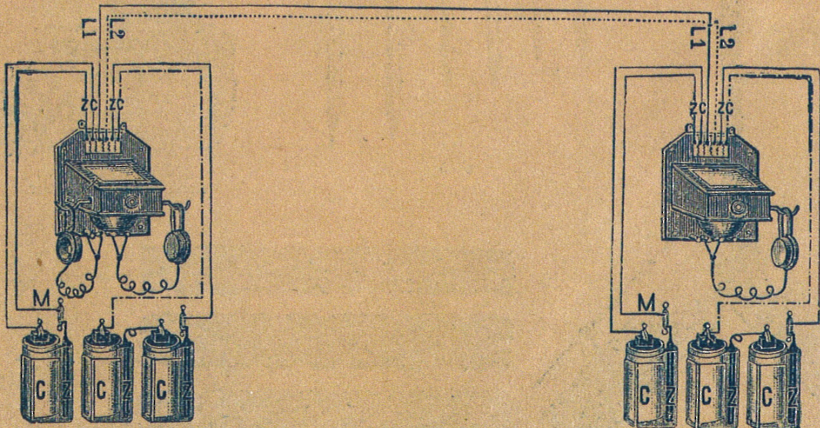
Az 5071—5076. sz. telefon-állomások gyakorlati alkalmazása. Praktische Anwendung der Telephon-Stationen No. 5071—5076.
