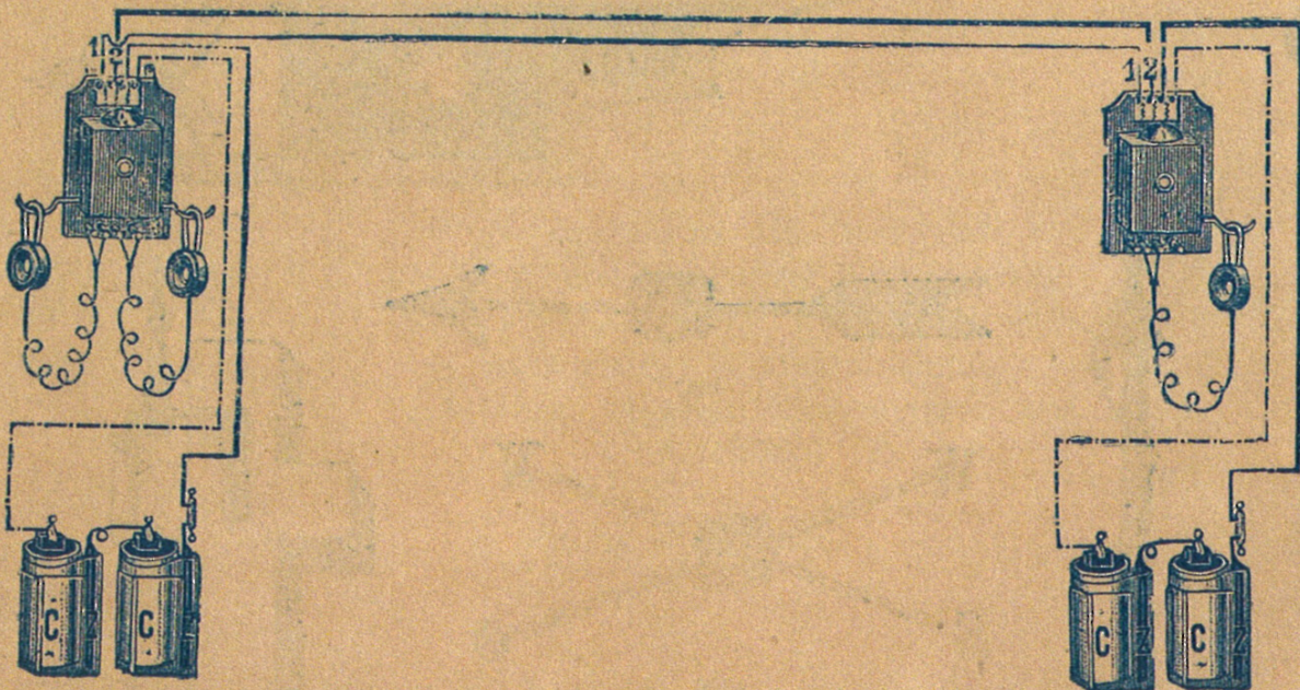
Az 5126—5131. sz. telefon-állomások gyakorlati alkalmazása. Praktische Anwendung der Telephon-Stationen No. 5126—5131.
