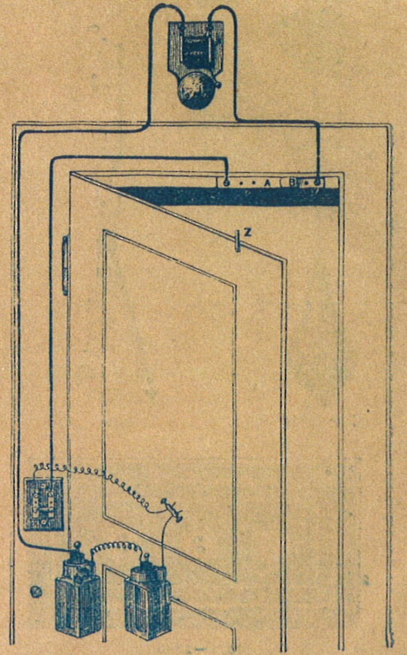
Az ajtóérintő gyakorlati alkalmazása. 1816. sz. Praktische Anwendung des Thürcontactes. Nr. 1816.
